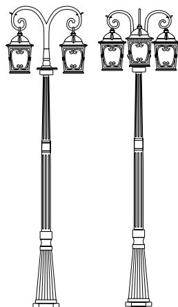
PL140 мощность: 3x100W высота: 2470мм
